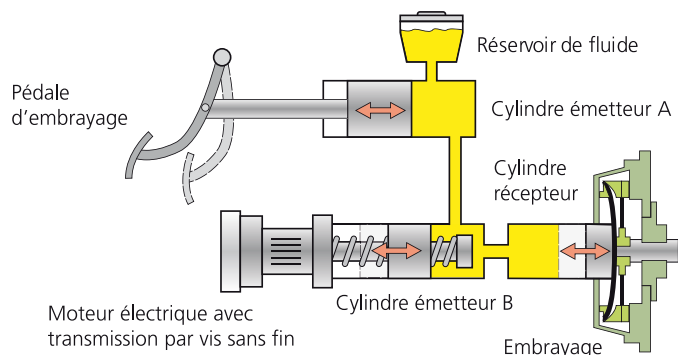
Fig. 2. Le concept d'actionnement de MTplus autorise aussi bien un actionnement classique via la pédale d'embrayage qu'un actionnement automatisé de l'embrayage via le moteur électrique avec transmission par vis sans fin.
