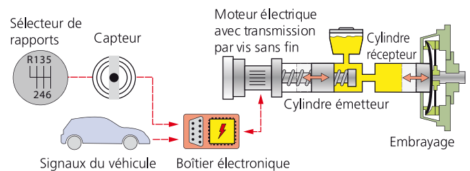
Fig. 5. L'EKM permet de renoncer totalement à une pédale d'embrayage.
