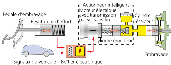
Fig. 3. Le système « clutch-by-wire » se passe de liaison directe entre la pédale d'embrayage et l'embrayage.
